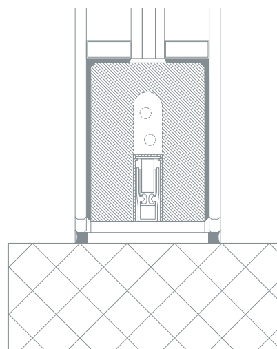
Vantail de porte EI30 bas
