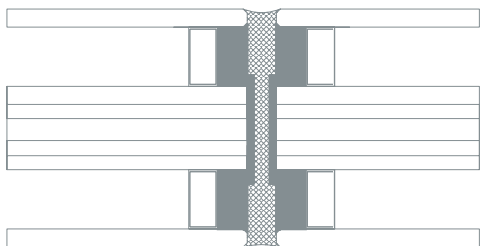
Joint entre deux vitrages fixes
