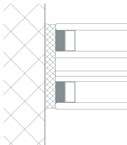
Raccord au mur vitrage fixe EI60
