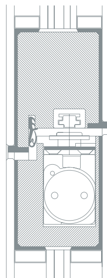
Vantail de porte EI30 haut
