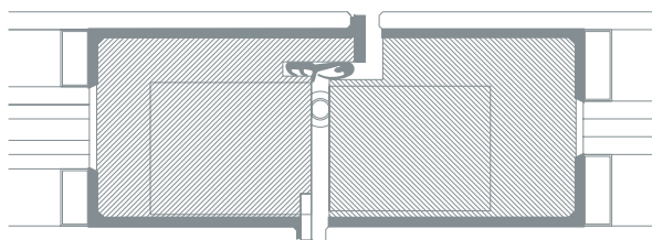
Raccord battant côté paumelles / vitrage fixe EI60
