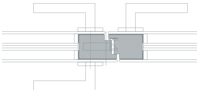
Partie centrale EI30 (2 vantaux)
