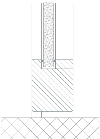
Raccordement au sol Porte Cristallo EI30
