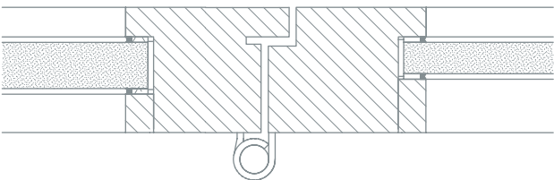
Raccordement porte Cristallo EI30 verre EI60
