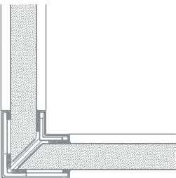
Angle 90° paroi Cristallo EI30 / EI60 avec profilé d'angle spécial Jegen thermostable (n° de brevet EP 2746519B1)
