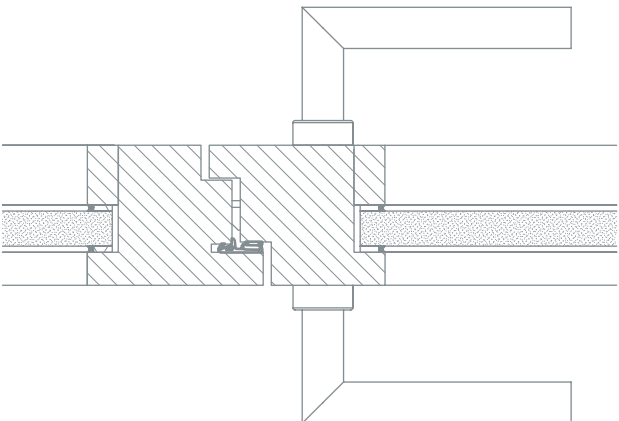
Partie centrale porte Cristallo 2 vantaux EI30
