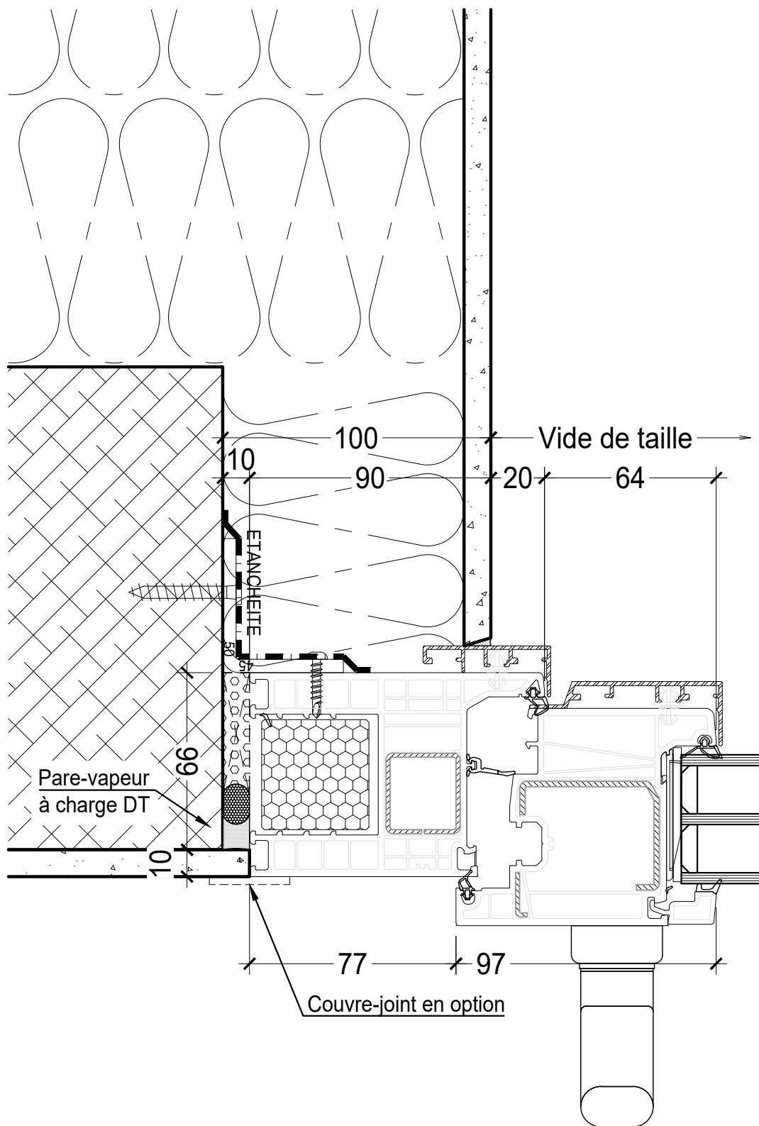
Concept du système d'étanchéité à charge DT
