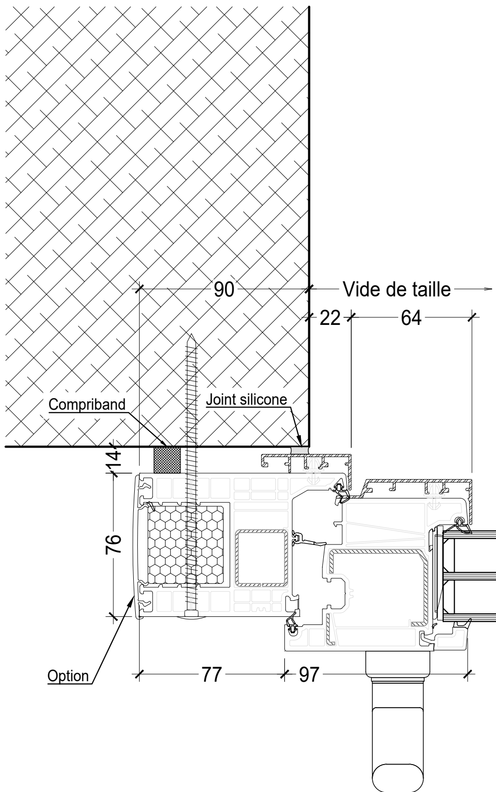
Concept du système d'étanchéité à charge DT
